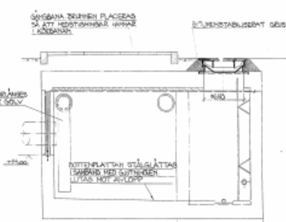
SEKTION C 5095 - 120
