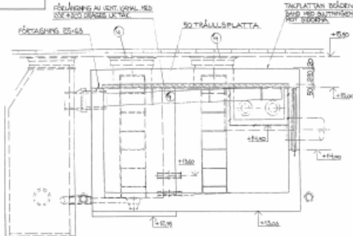
SEKTION B 5095 - 120
